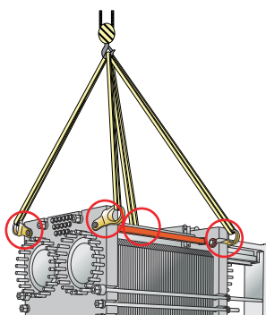
Рис. 7: Подъемное устройство для T50. Требуется крепежное оборудование.
