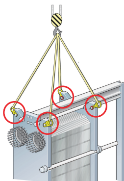
Рис. 6: Подъемное устройство для T45, TL35 и WideGap 350. Крепежное оборудование не требуется.
