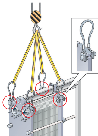
Рис. 5: Подъемное устройство для T35 и TS35. Требуется крепёжное оборудование.
