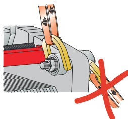
Рис. 8: Подъемное устройство для TS50. Используйте четыре внутренние проушины для подъема пластинчатого теплообменника. ЗАПРЕЩАЕТСЯ использовать крепежные точки, предназначенные для транспортирования! Требуется крепежное оборудование.
